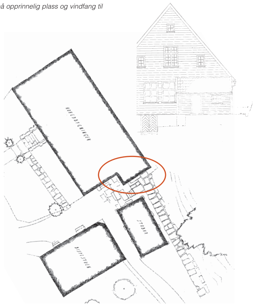
Plantegning og fasade av vindfanget på nordsiden av Hovedhuset, oppmålt av arkitekt Per Grieg 1927
